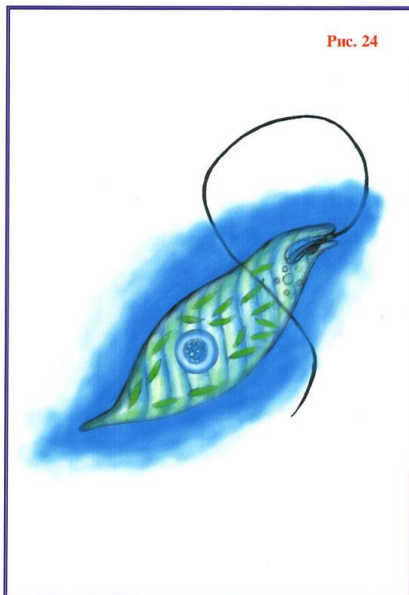
Fig. 24. Green Euglena.
